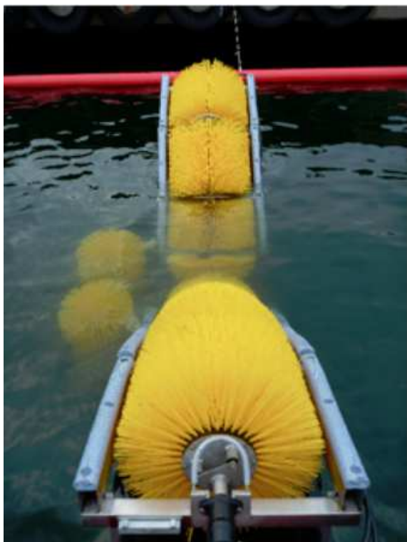
Detalj av borttvätt som visar hur borstarna är konstruerade
